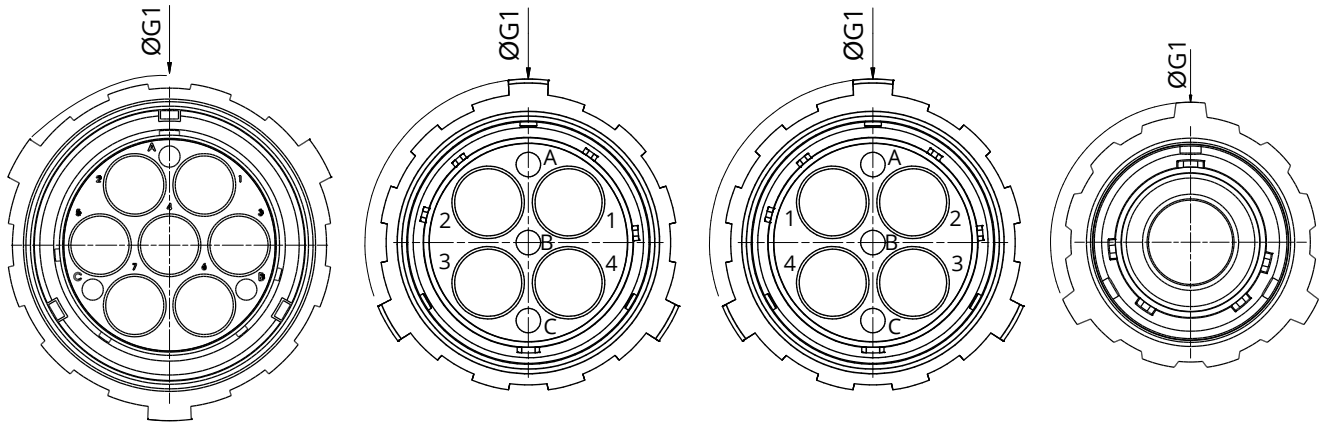
Size 48 and module n° A7/I7
